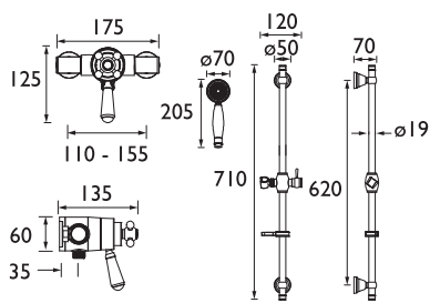
Riser Kit
